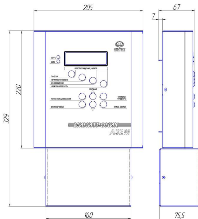
Рис.2а. Габаритный чертеж и установочные размеры АПКП и ВПУ.
