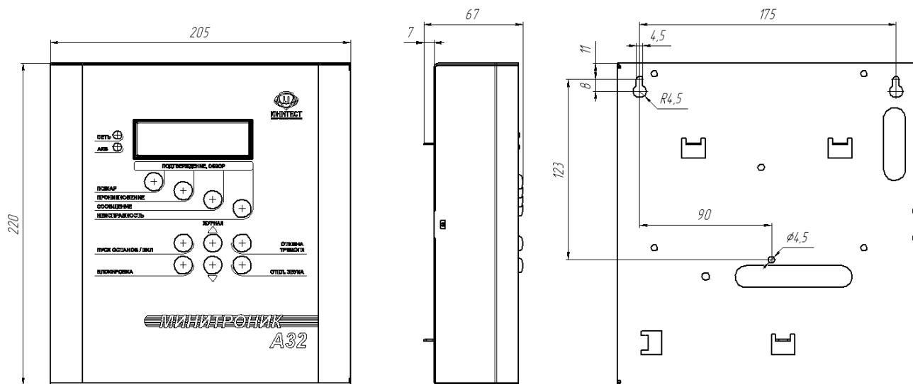
Рис.2а. Габаритный чертеж и установочные размеры АПКП и ВПУ.
