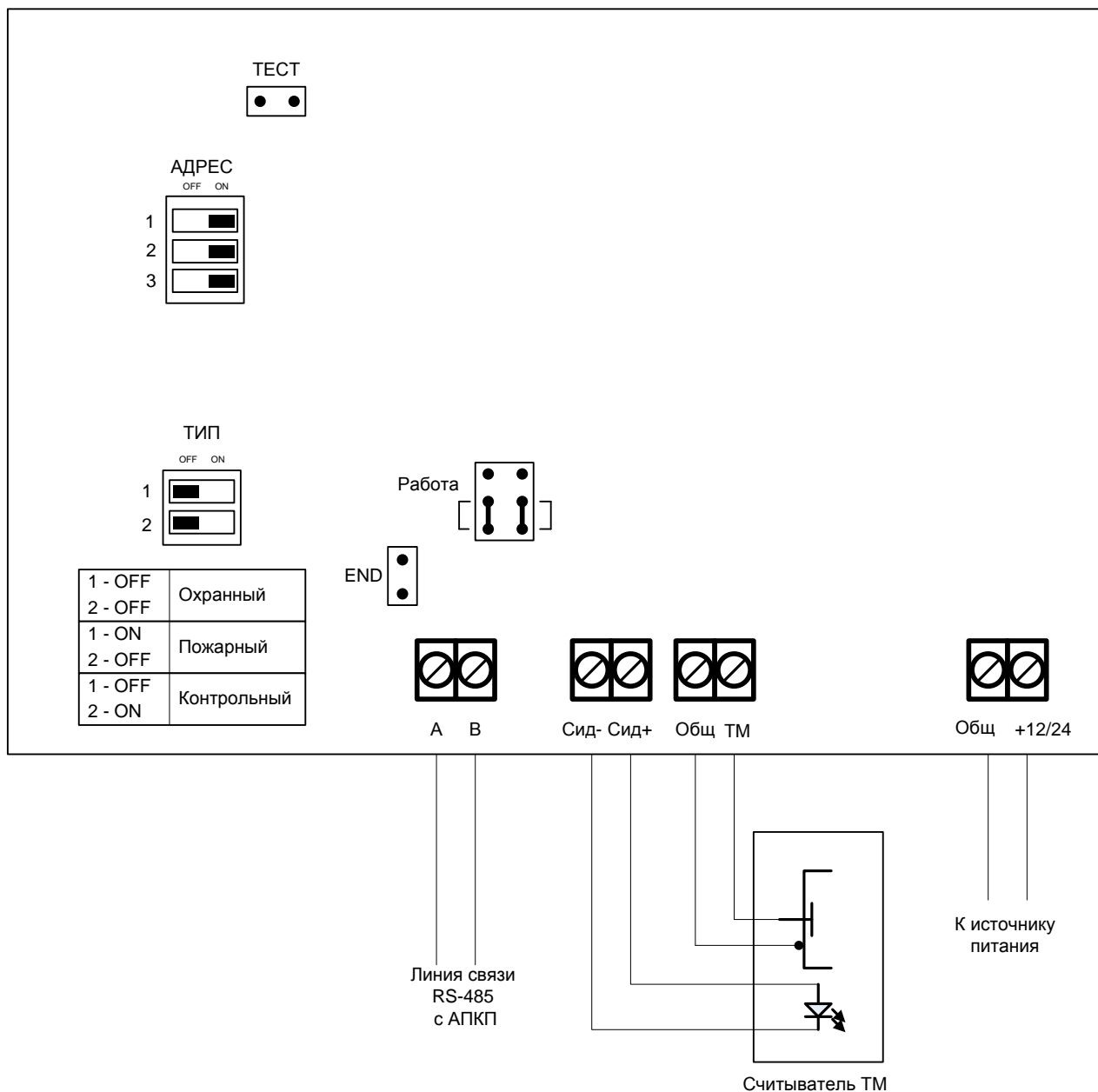
Рис.3. Расположение клемм подключения на плате индикации СДИ
